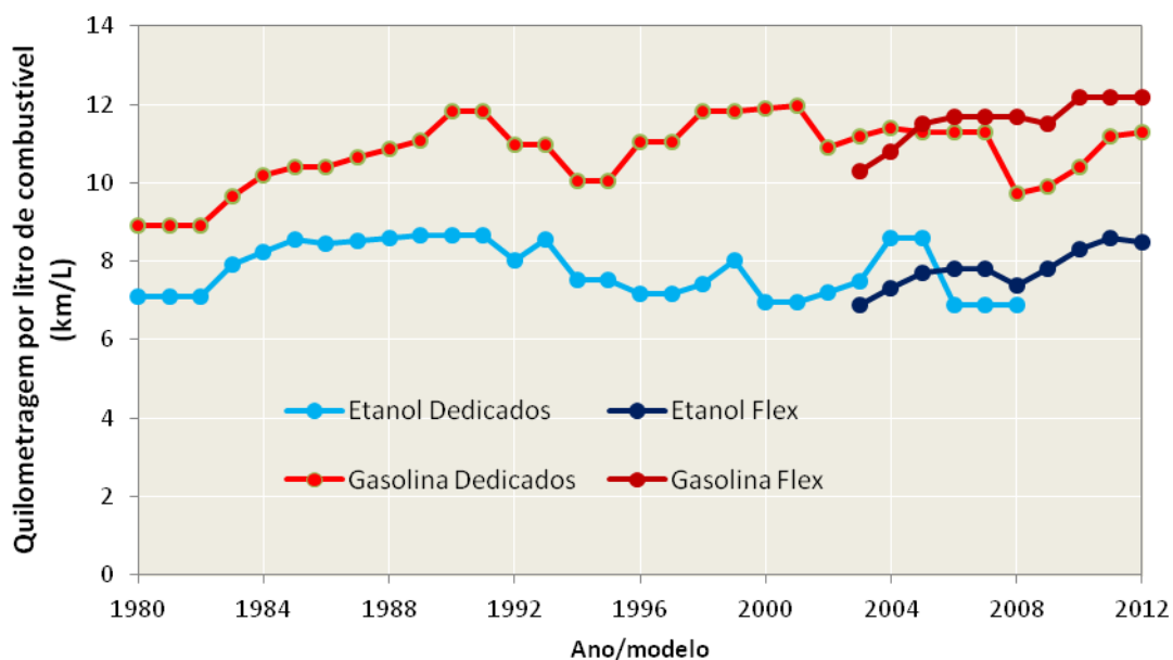
Gráfico 13: Quilometragem por litro de combustível para automóveis
